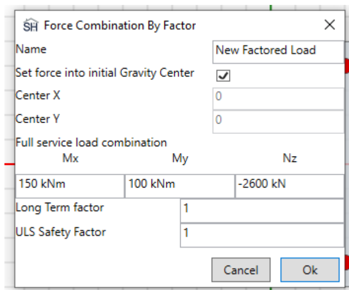
Рисунок 3-41. Характеристики загрузки
