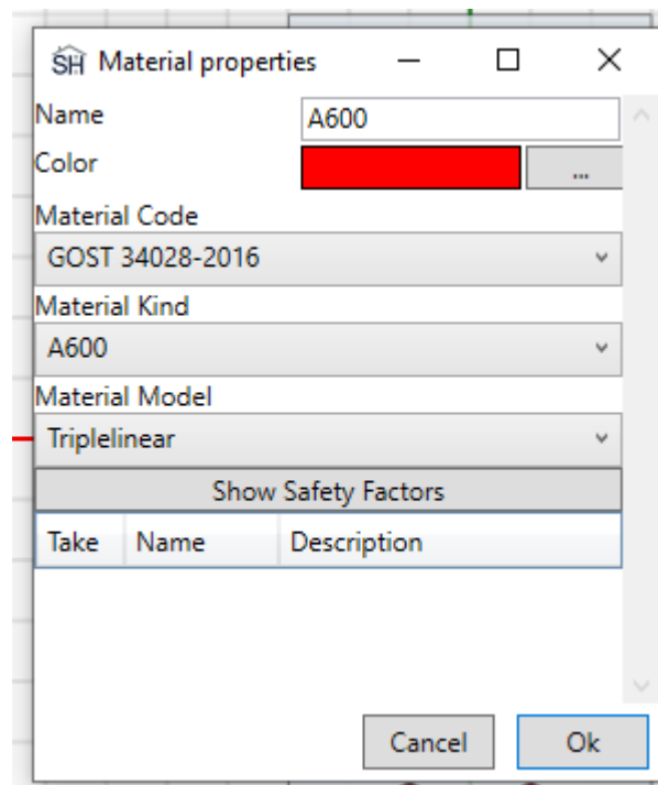
Рисунок 3-47. Материал арматуры
