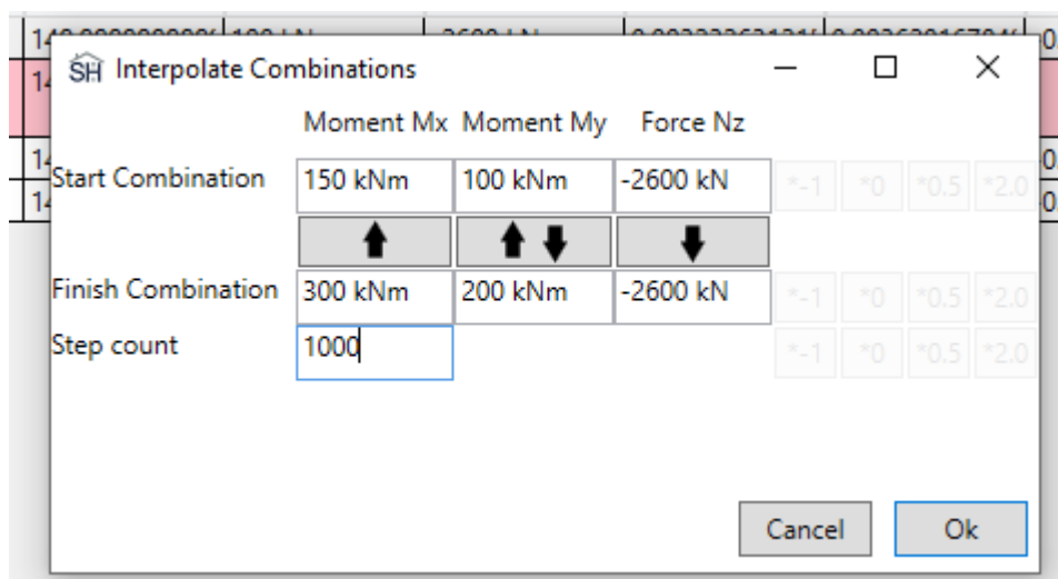
Рисунок 3-43. Ввод данных для интерполяции усилий при постоянной продольной силе
