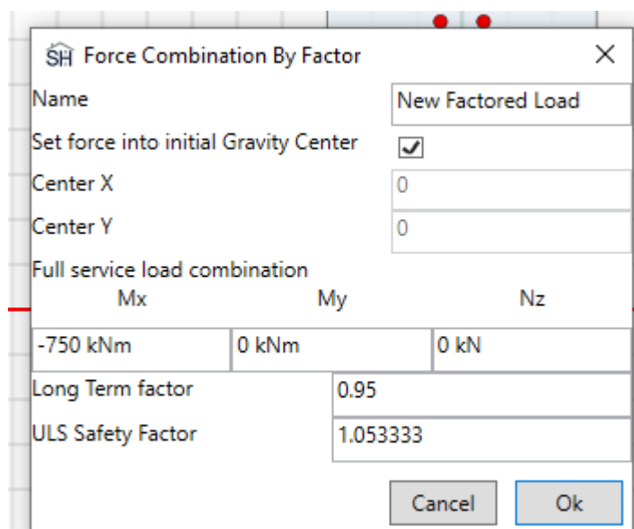
Рисунок 3-56. Свойства загрузки
