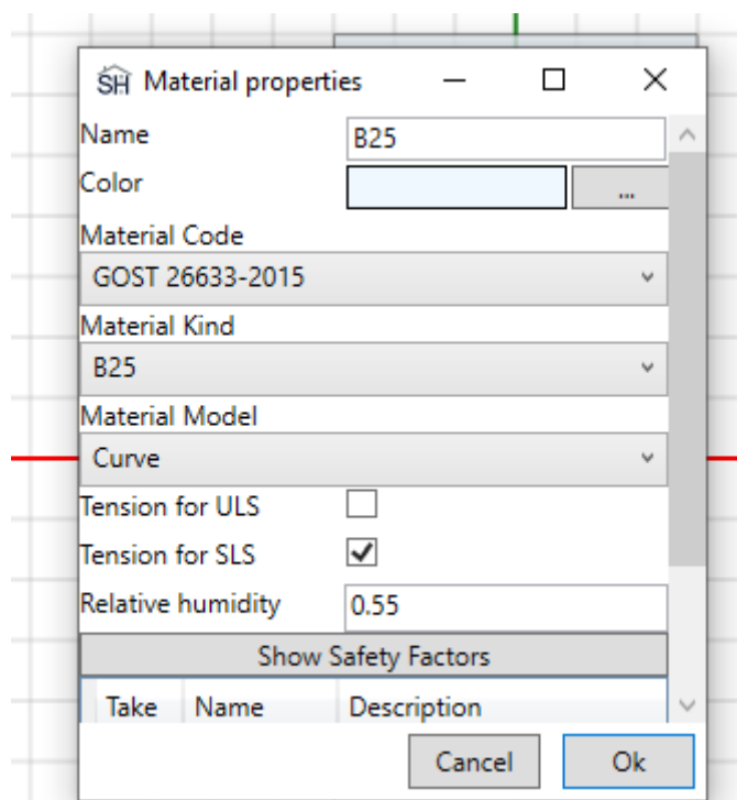
Рисунок 3-46. Материал бетона Зададим материал для арматуры
