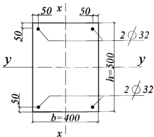
Рисунок 3-37. Расчетное сечение элемента по данным источника Зададим материал для бетона
