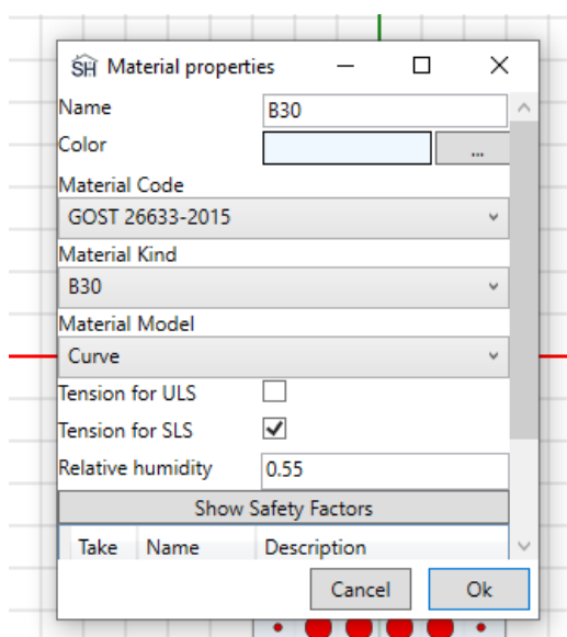
Рисунок 3-54. Материал бетона
