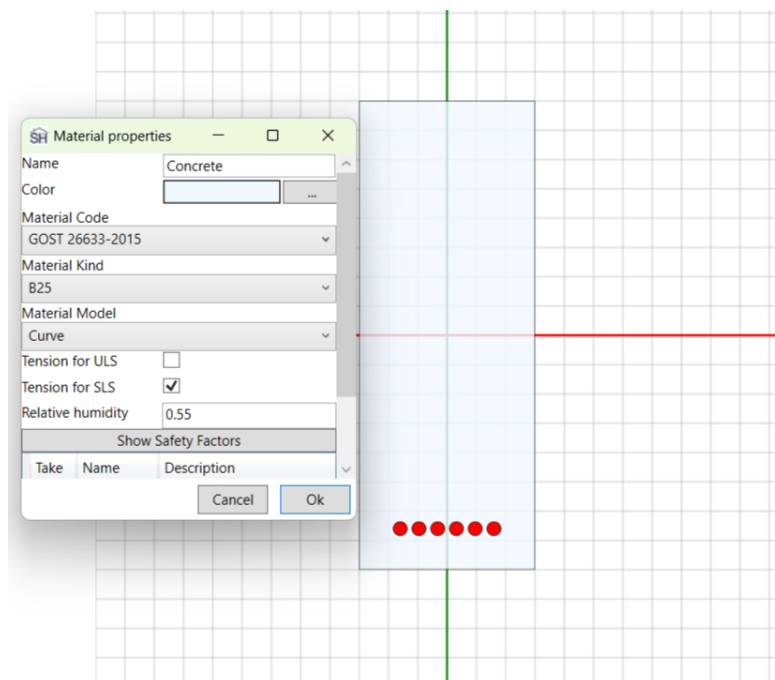
Рисунок 3-2. Материал бетона
