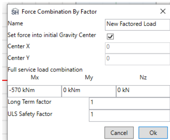
Рисунок 3-48. Ввод данных по загрузению
