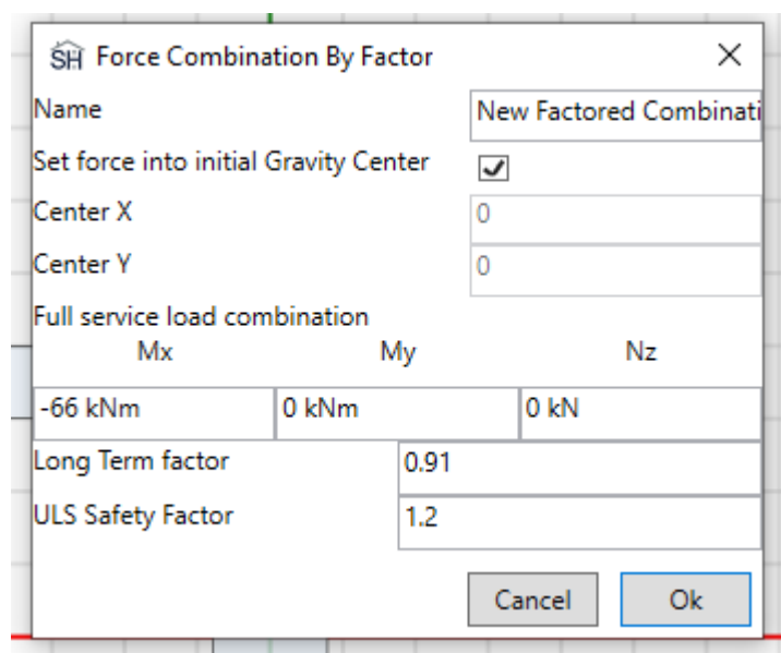
Рисунок 4-27. Ввод данных по загрузению
