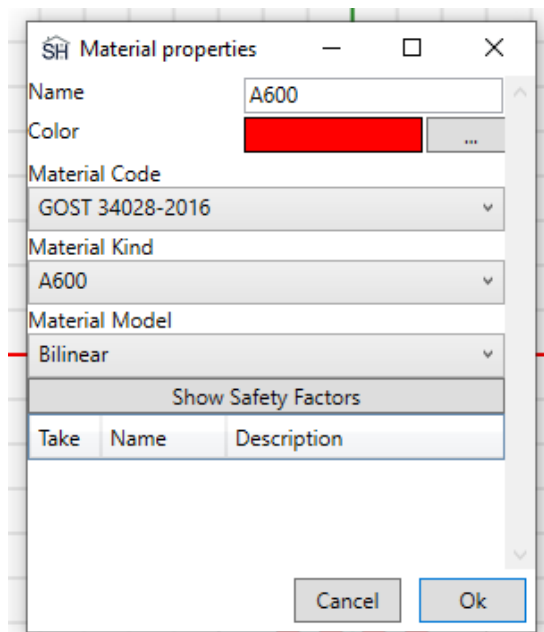
Рисунок 3-55. Материал арматуры.
