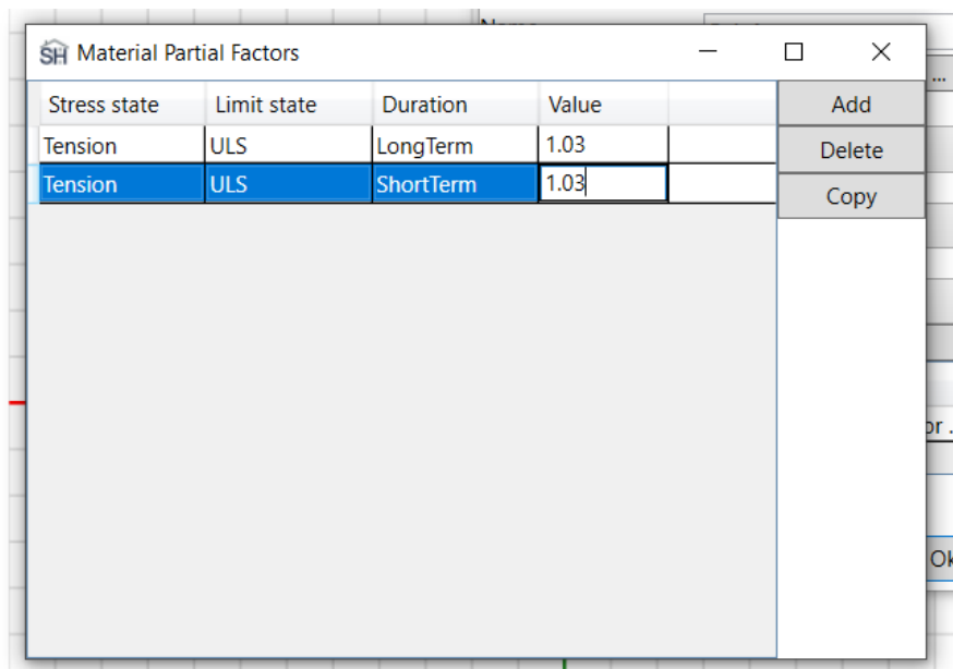
Рисунок 3-40. Ввод дополнительного коэффициента условий работы для арматуры Зададим комбинацию нагрузок
