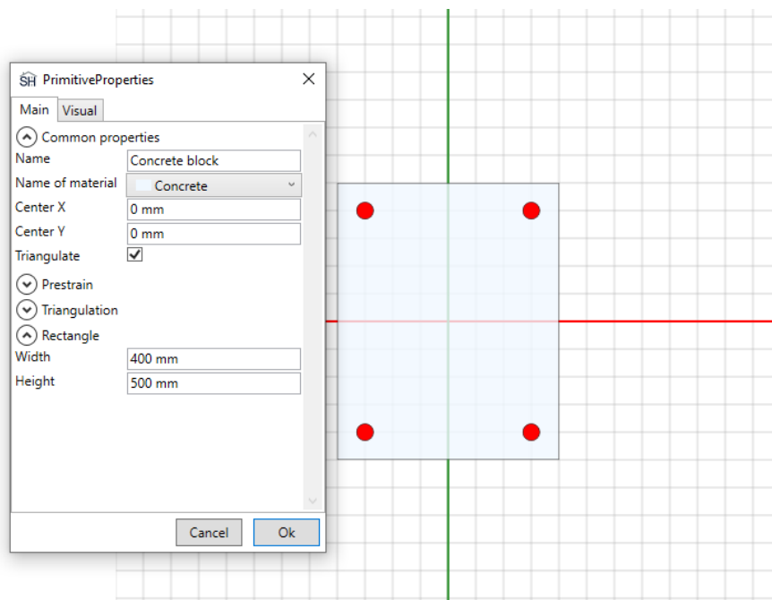
Рисунок 3-36. Расчетное сечение элемента в StructureHelper
